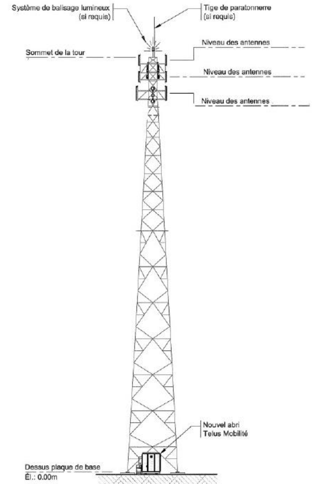
ÉLÉVATION DE LA TOUR TOUR AUTOPORTANTE
